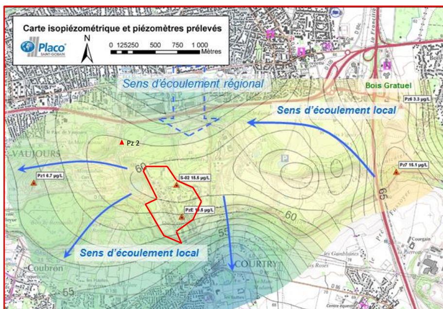
Figure 5 - Carte isopiezométrique et piézomètres prélevés
